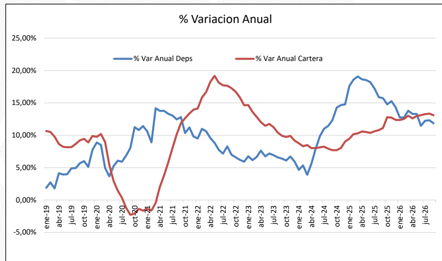
Variación anual
