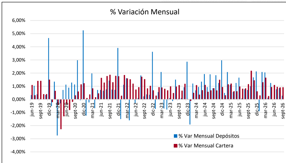
Variación mensual
